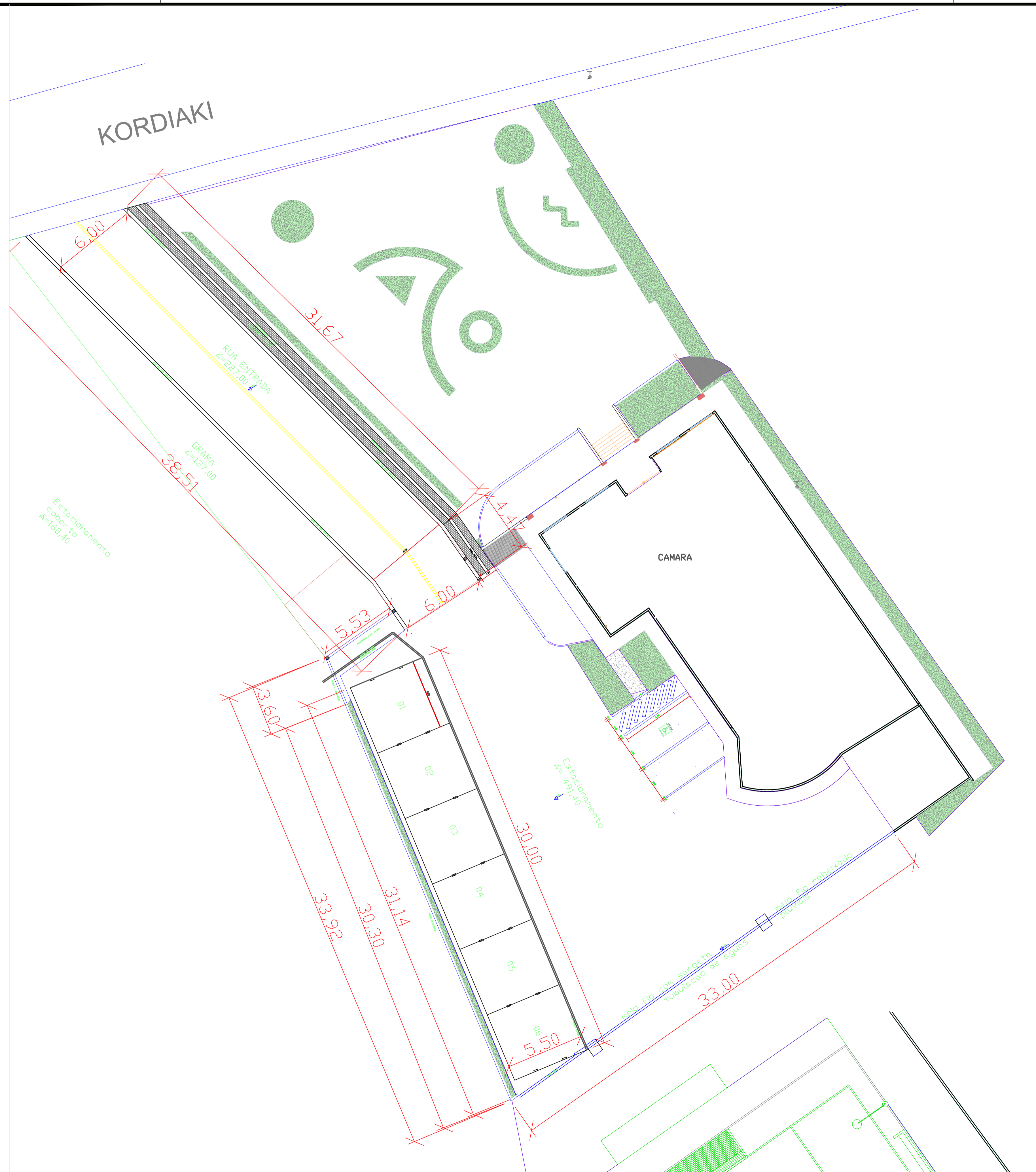
PLANTA DE IMPLANTAÇÃO
